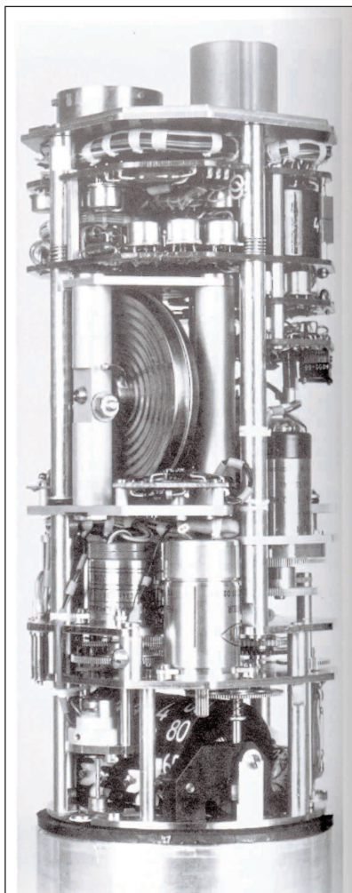
Altimètre à aiguille et à tambour de Concorde Jaeger (1974) (Source Gifas).
