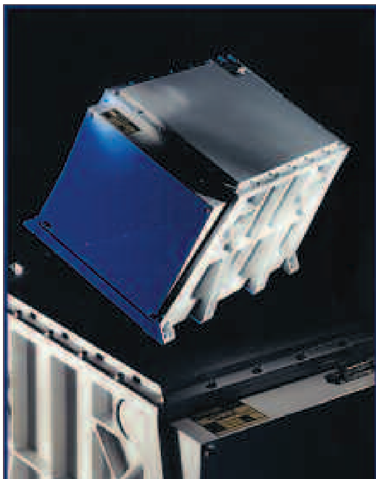
Centrale Quasar Thales (Source Thales).
