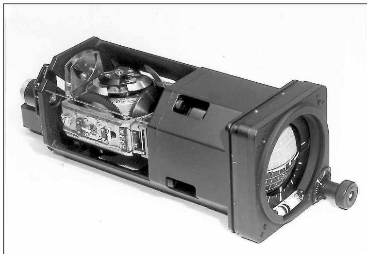
Horizon gyroskopique SFENA 800 (Horizon de secours) (Source SFENA).
