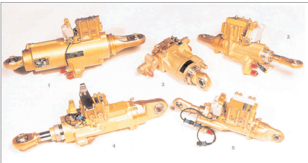
Les servocommandes de l'Airbus A 300 (Air Equipement) (Source GIFAS). 1 : Direction, 2 : Profondeur, 3 : Spoilers aérofrens, 4 : Ailerons toutes vitesses, 5 : Ailerons basses vitesses.
